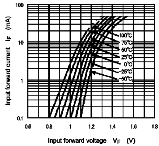
Fig. 11.4 I_F - V_F
