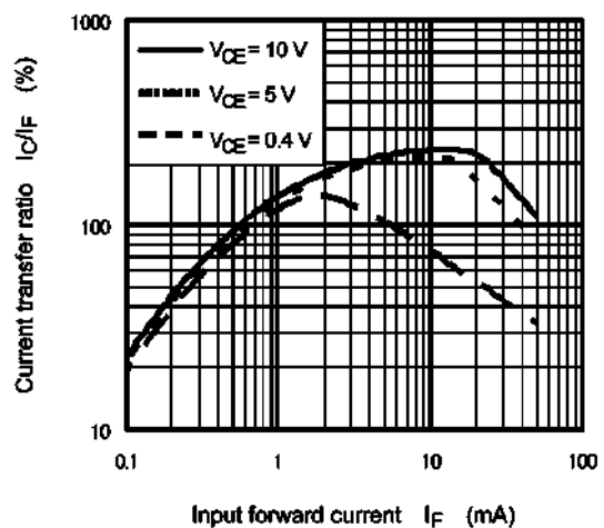
Fig. 11.11 I_C/I_F - I_F
