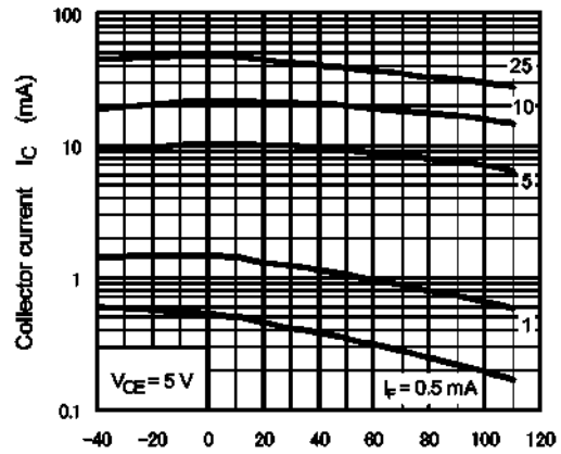
Fig. 11.13 I_C - T_a
