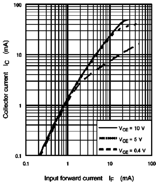
Fig. 11.9 I_C - I_F
