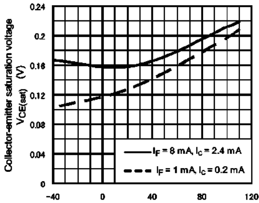
Fig. 11.12 V_{CE(sat)} - T_a
