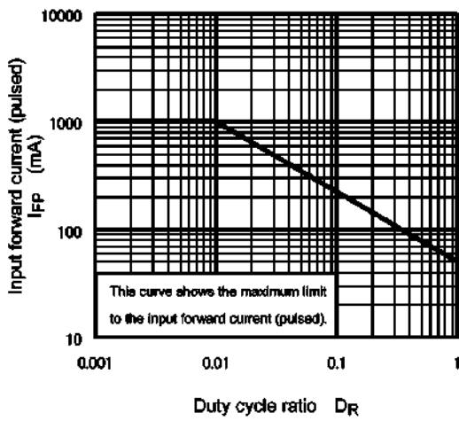
Fig. 11.3 I_{FP} - D_R
