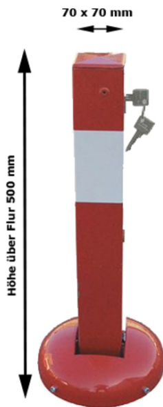
Technische Ansicht:
