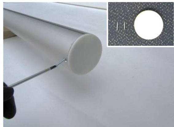
Montage Pfostenverschlusskappe runder Pfosten:
