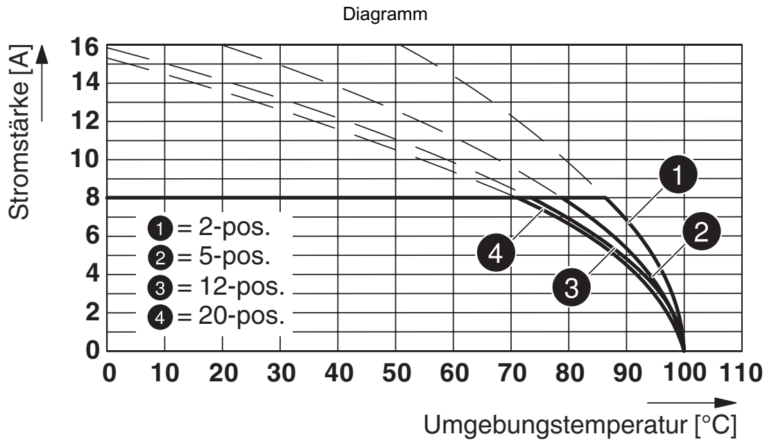
Typ: FRONT-MC 1,5/...-ST-3,81 mit MCV 1,5/...-G-3,81
