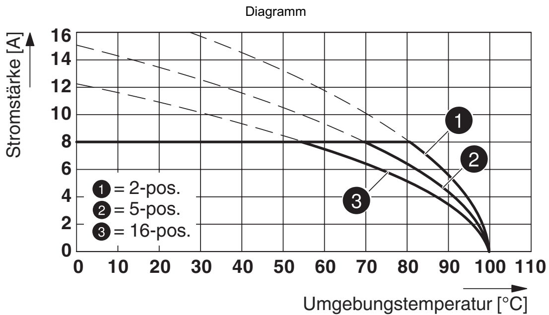
Typ: FRONT-MC 1,5/...-ST-3,81 mit MCDV 1,5/...-G1-3,81
