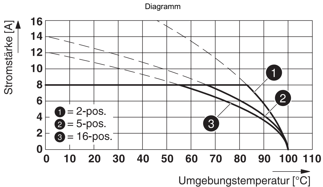
Typ: FRONT-MC 1,5/...-ST-3,81 mit MCD 1,5/...-G1-3,81
