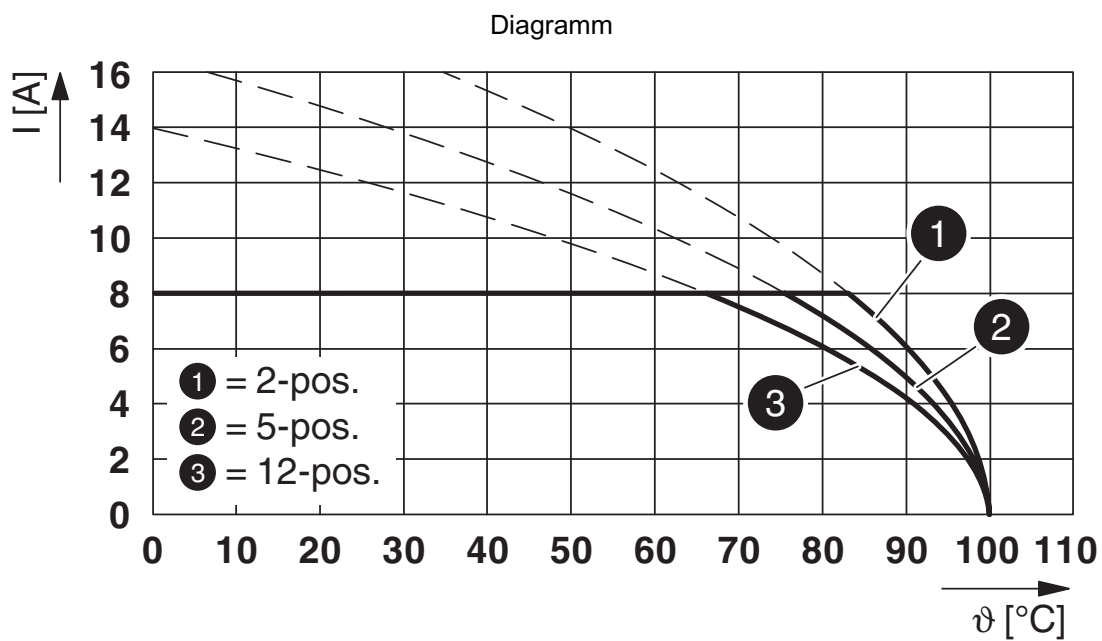
Typ: FRONT-MC 1,5/...-ST-3,81 mit MC 1,5/...-G-3,81 P... THR
