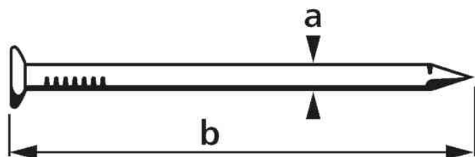
Visuel de référence: pointe, tête fraisée, pictogramme
