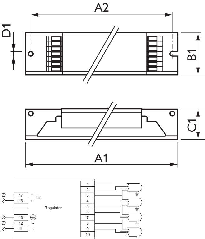
HF-R 4 lamps TL5/PL-L/TL-D
