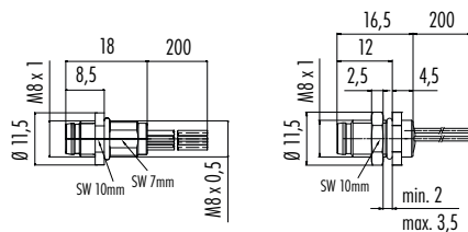
von hinten verschraubbar
