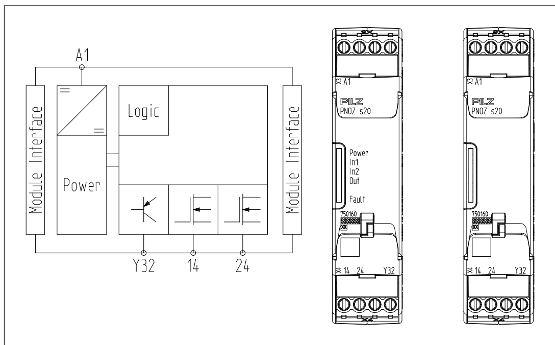
Abb.: Mitte: Frontansicht mit Abdeckung, rechts: Frontansicht ohne Abdeckung
