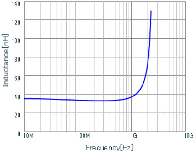
LQP03HQ33NJ02 L.
