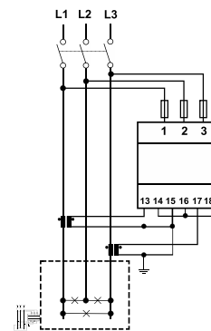
Fig. 7 Dreiphasig ohne Nulleiter (3-drahtig). MID
