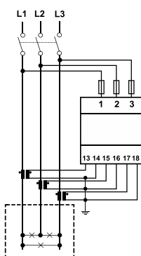
Fig. 6 Dreiphasig ohne Nulleiter (3-drahtig). MID
