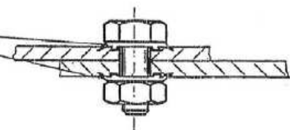
Auflagefläche für Schraubenkopf- bzw. Mutter gerillt bearing surface for screw head- or nut grooved
