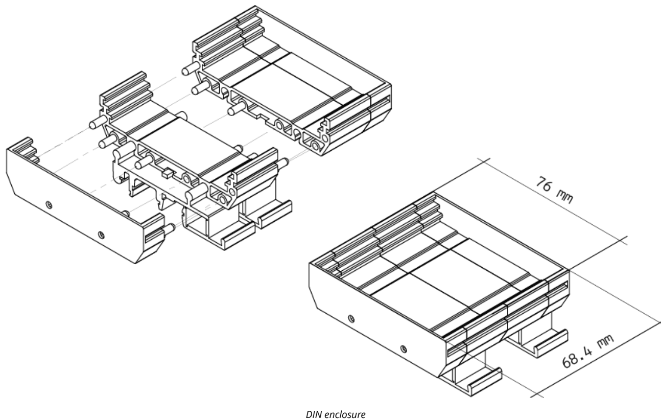
DIN enclosure
