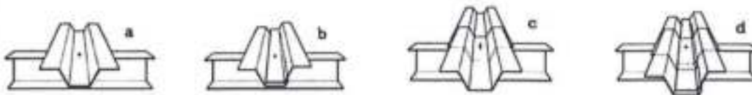
Verbindung mit einem Einzblock Verbindung mit einem Längsstoß Verbindung mit einem Querstoß Verbindung mit einem Längs- und Querstoß
