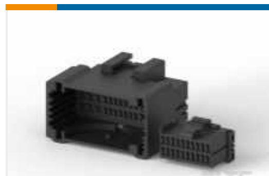
TE Teilnr.:174967-2 MULTILOCK, STECKVERBINDERGEHÄUSE
