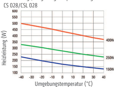
Heizleistung-/Umgebungstemperatur-Diagramm
