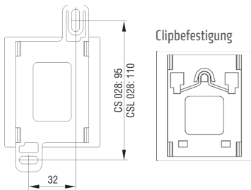
Ansicht Rückseite Schraubbefestigung
