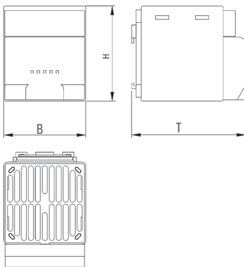
Ansicht Rückseite Schraubbefestigung
