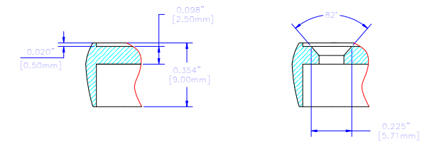
SECTION A-A SCALE 2:1
