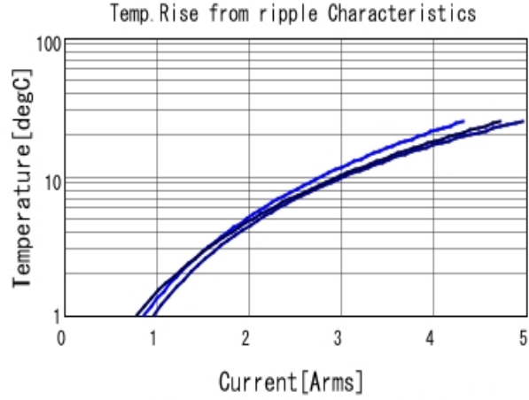
KCM55WR72A156MH01 Temp. rise ■ 50kHz ■ 100kHz ■ 300kHz
