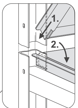
Planoflex Verbinder Anbau 3000
