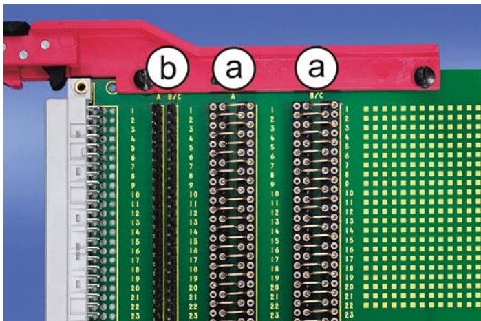
a: Messfeld für Strom- und Spannungsmessung b: Stiftleiste für Wire Wrap
