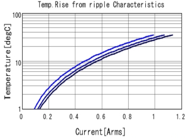
GRM033C81E104ME14 Temp. rise ■ 400kHz ■ 800kHz ■ 1MHz
