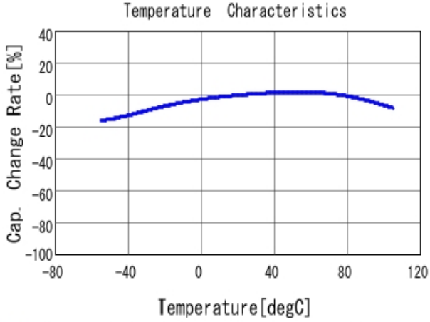
■ GRM033C81E104ME14 C-Temp. capchange, DCO. 0V, ACO. 2V rm
