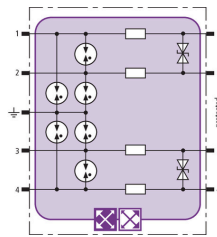
Prinzipialschaltbild BXT ML4 BD EX 24
