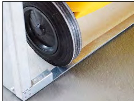
Zum absolut leichtgängigen Einstellen und Herausfahren auch von vollen Mülltonnen wird das Bodenprofil im Türbereich ausgespart.
