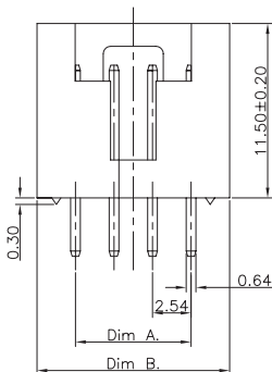
(4~18 Pin)
