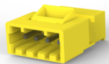
TE Teilenummer 3-641436-4 04P MTA156 CONN ASSY LF
