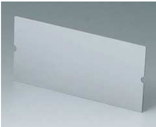
A9195201 Frontplatte Aluminium matt eloxiert 113x58x1mm
