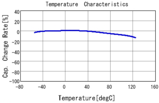
■ GCJ31CC72A225KE01 C-Temp. capchange, DCO. 0V, AC1. 0V rm
