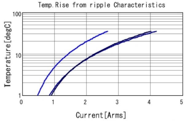
GCJ31CC72A225KE01 Temp. rise ■ 100kHz ■ 500kHz ■ 1MHz
