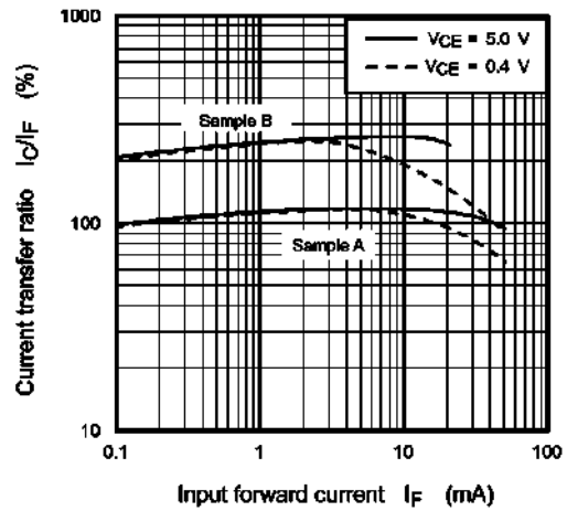
Fig. 11.10 I_C/I_F - I_F
