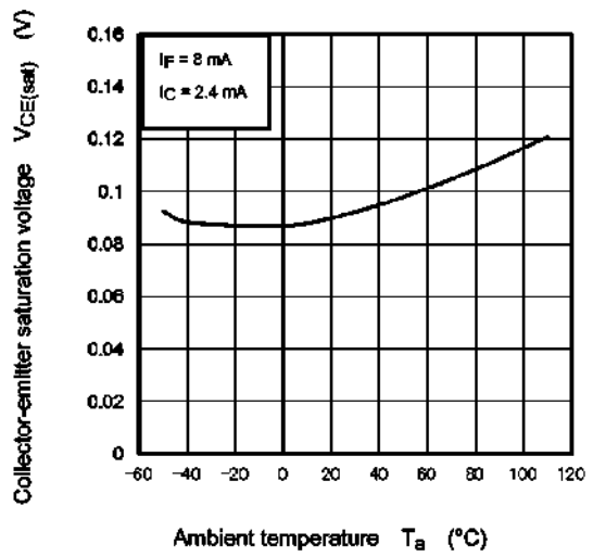
Fig. 11.12 V_{CE(sat)} - T_a
