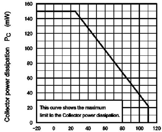
Ambient temperature T_a (°C) Fig. 11.2 P_C - T_a
