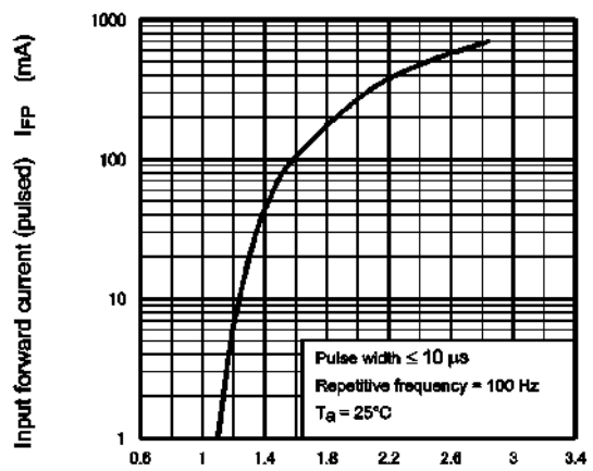
Fig. 11.6 I_{FP} - V_{FP}
