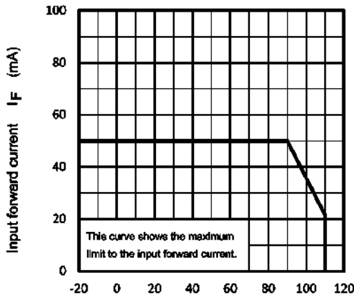
Ambient temperature T_a (°C) Fig. 11.1 I_F - T_a
