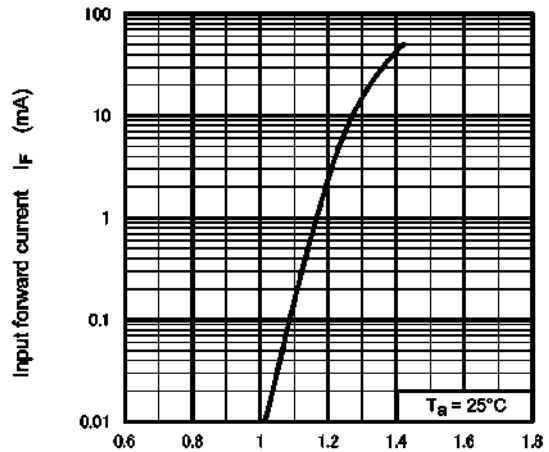
Fig. 11.4 I_F - V_F
