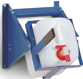
Abfüllbock AB 10-L, zur Wandmontage und als Standgerät geeignet, Bestell-Nr. 136-492-J0
