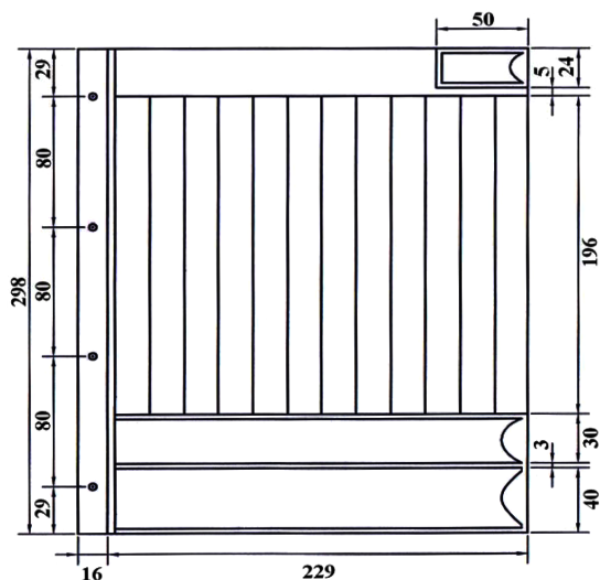
Dimensions : Millimetres
