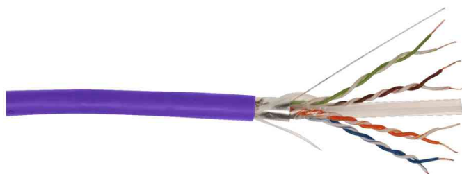
Câble d'installation cat.6, F/UTP, LSOH
