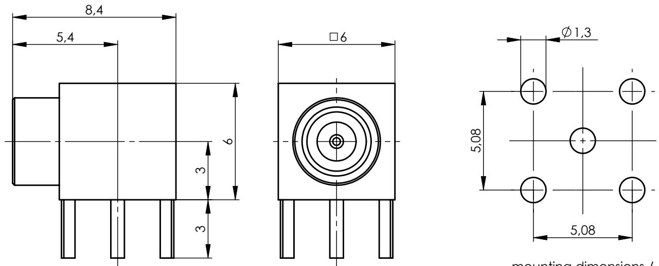
mounting dimensions / Einbaumaße Z025
