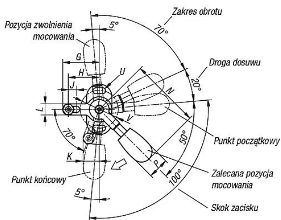
Wykonanie prawostronne
