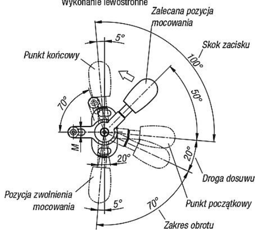
Wykonanie lewostronne
