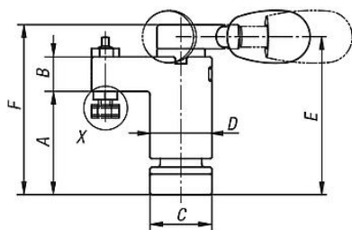
Wykonanie prawostronne
