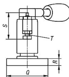
Wykonanie lewostronne
