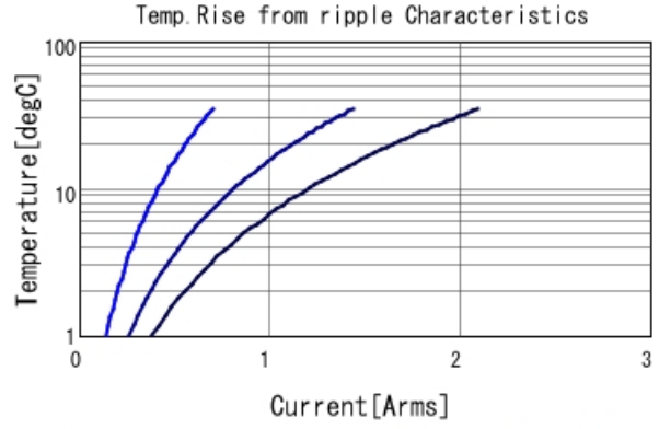
GRM43DR72E334KW01 Temp. rise ■ 30kHz ■ 100kHz ■ 300kHz
