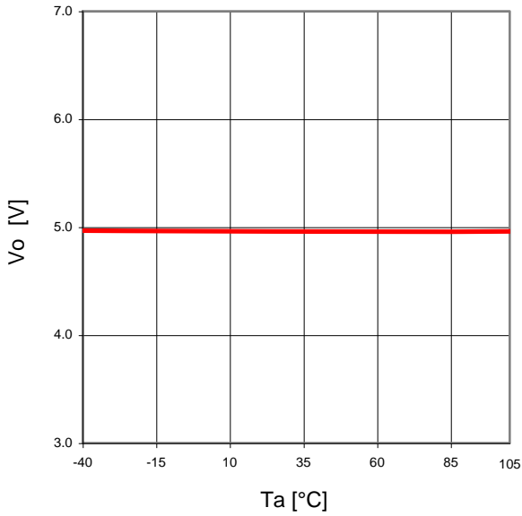
Fig.21 Ta-Vo (Io=0mA)
