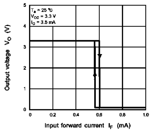
Fig. 12.2.12 V_O - I_F
