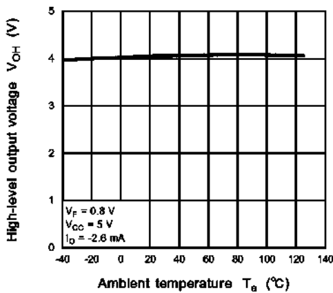
Fig. 12.2.5 V_{OH} - T_a
