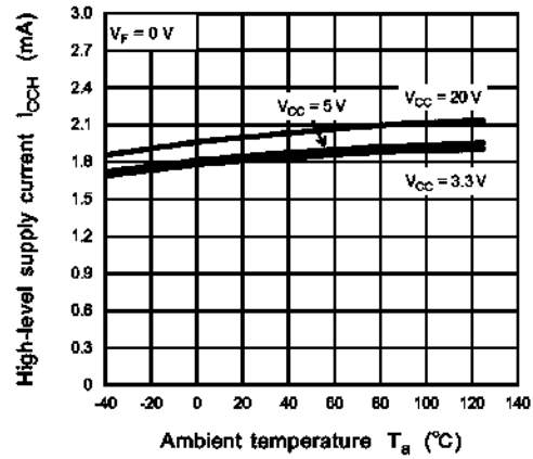
Fig. 12.2.8 I_{CCH} - T_a
