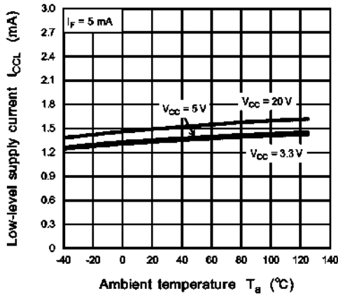
Fig. 12.2.7 I_{CCL} - T_a
