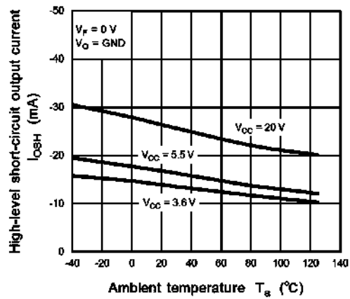
Fig. 12.2.10 I_{OSH} - T_a
