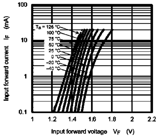
Fig. 12.2.1 I_F - V_F
