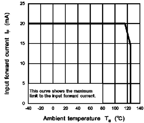
Fig. 12.2.2 I_F - T_a
