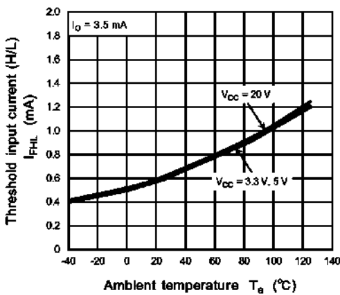
Fig. 12.2.11 I_{FHL} - T_a
