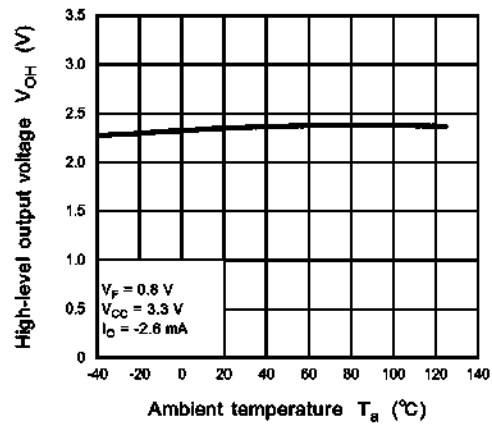
Fig. 12.2.4 V_{OH} - T_a
