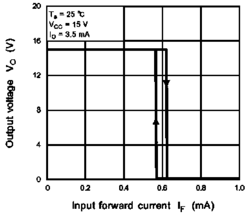
Fig. 12.2.13 V_O - I_F
