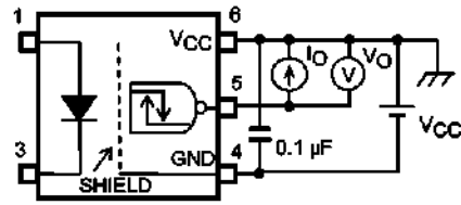
Fig. 12.1.2 V_{OH} Test Circuit
