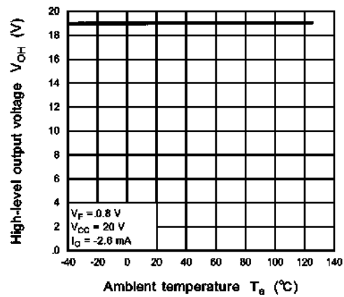
Fig. 12.2.6 V_{OH} - T_a
