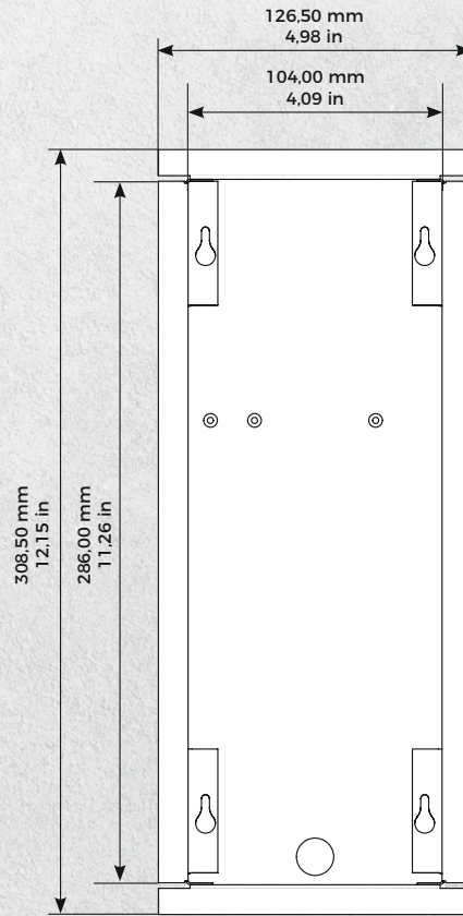
Montagerückgehäuse
