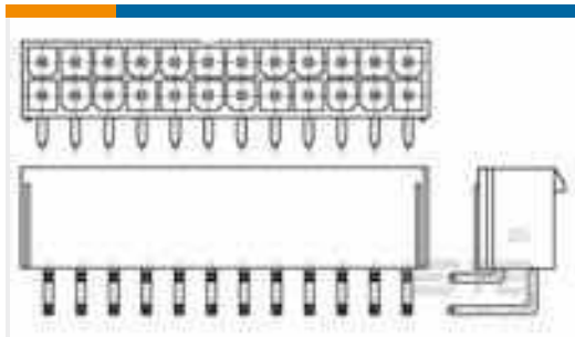
TE Teilnr.:1-1586041-4 14P VAL-U-LOK R/A HDR V2
