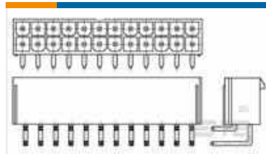
TE Teilnr.:1-1586041-2 12P VAL-U-LOK R/A HDR V2
