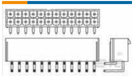
TE Teilnr.:1586041-8 8P VAL-U-LOK R/A HDR V2
