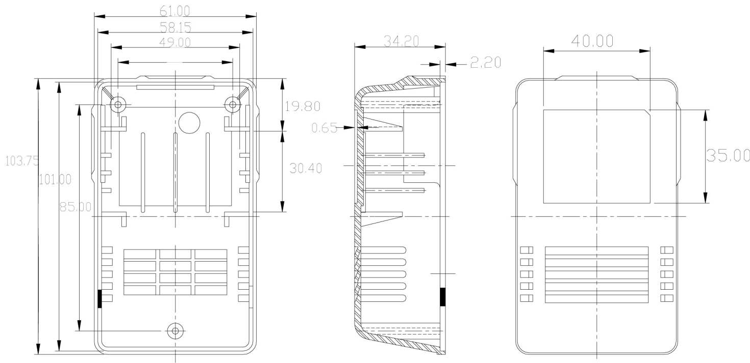
Base (pins)
