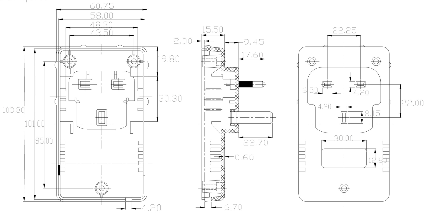
Base (pins)
