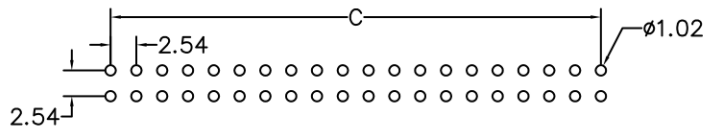
Leiterplattenbohrbild
