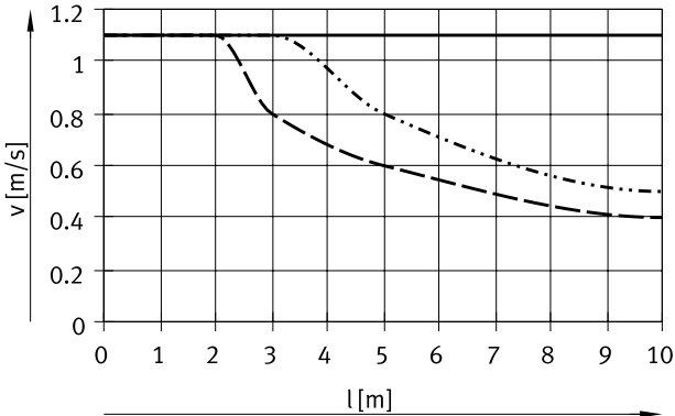
Für Baugröße 32
