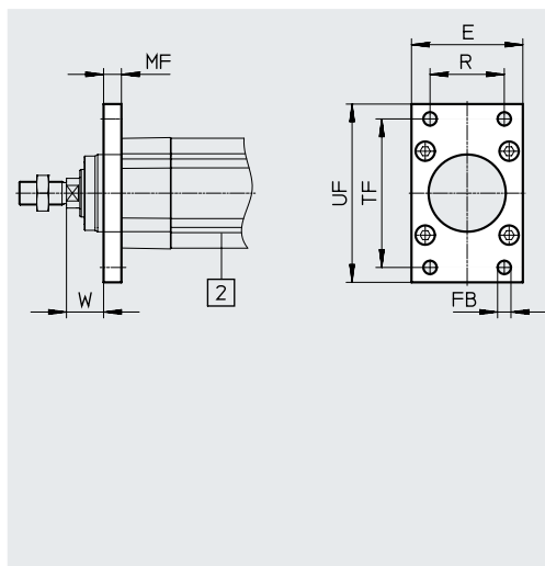
[2] Elektrozyylinder ESBF
