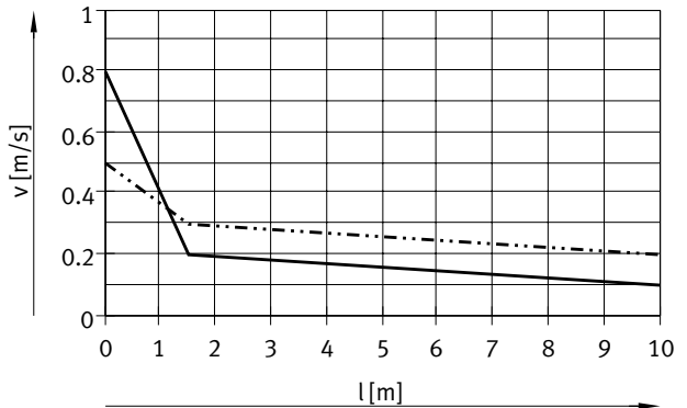
Für Baugröße 63
