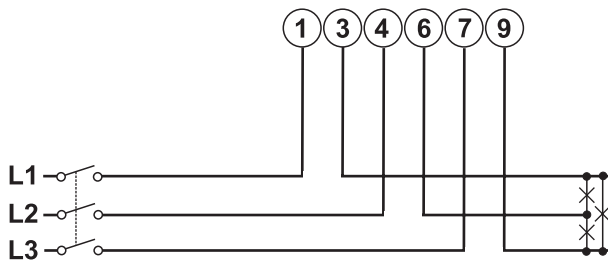
Fig. 33 AV2
