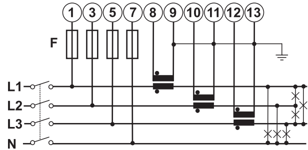
Fig. 32 AV5
