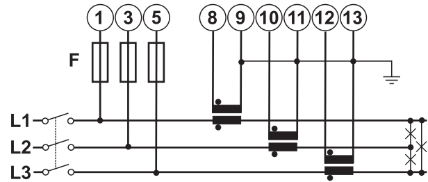
Fig. 34 AV5
