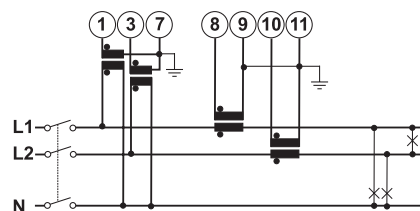
Fig. 17 AV6
