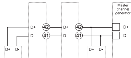
Fig. 30 Dupline port
