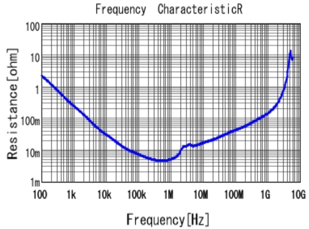
■ GCJ31CR71A226KE01 R DCOV, 25degC
