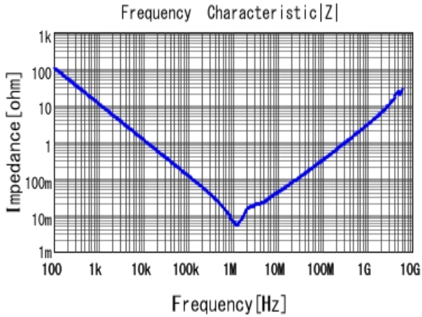
■ GCJ31CR71A226KE01 |Z| DCOV, 25degC
