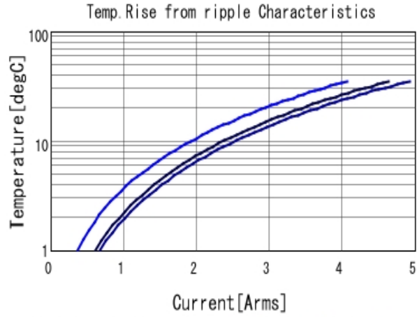
GCJ31CR71A226KE01 Temp. rise ■ 80kHz ■ 400kHz ■ 800kHz
