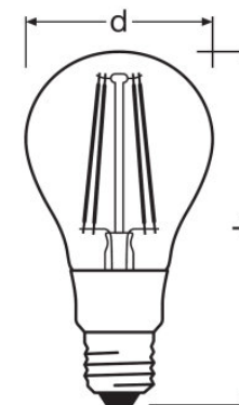
P RF CLAS A 95 12 W/827 E27
