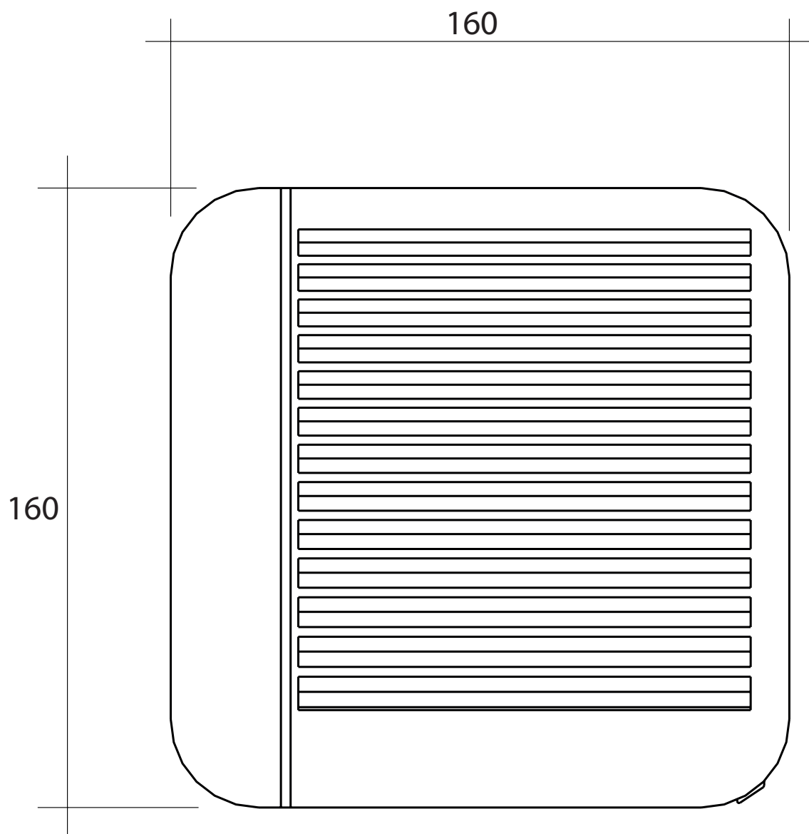
Zentrifugallüfter FLUX 100 Timer/Hygro Material: Kunststoff
