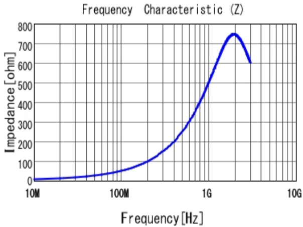
■ LQW18CA85NJ00 |Z|
