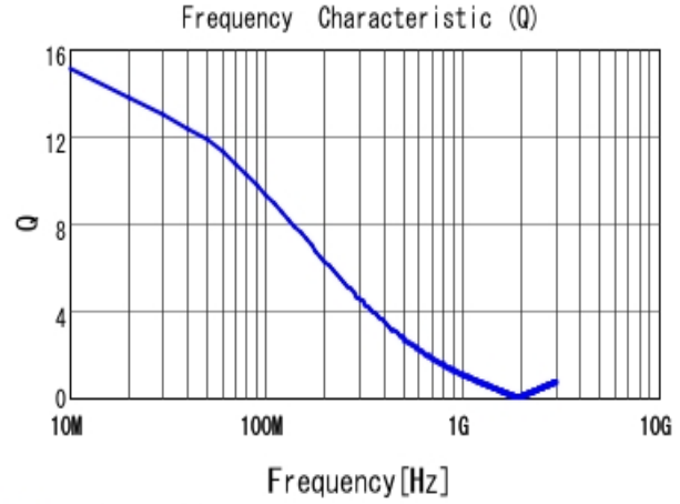
■ LQW18CA85NJ00 Q
