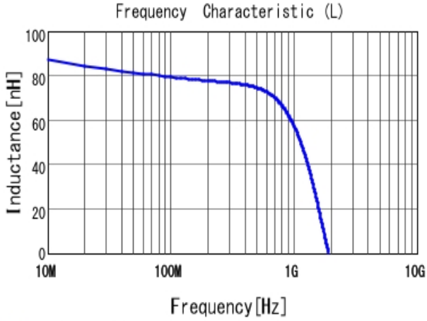
■ LQW18CA85NJ00 L
