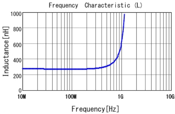
■ LQW18ANR27G80 L
