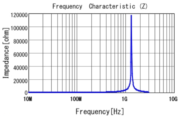
■ LQW18ANR27G80 |Z|
