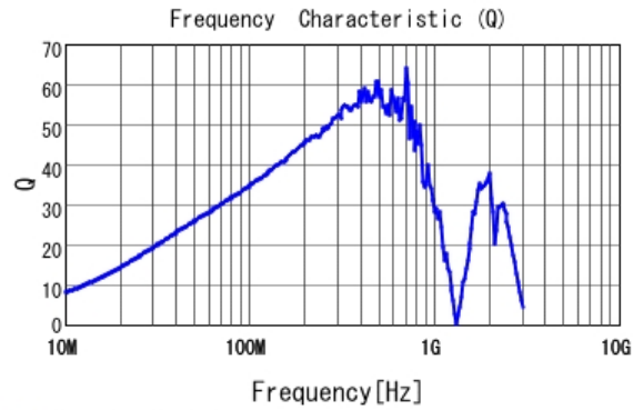
■ LQW18ANR27G80 Q
