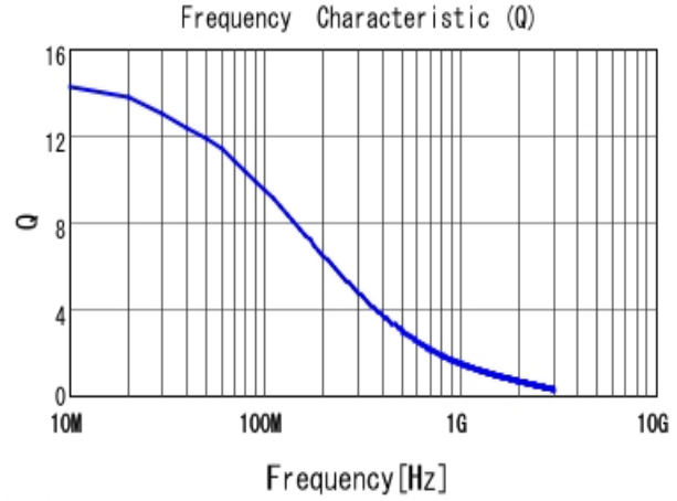
■ LQW18CA32NJ00 Q
