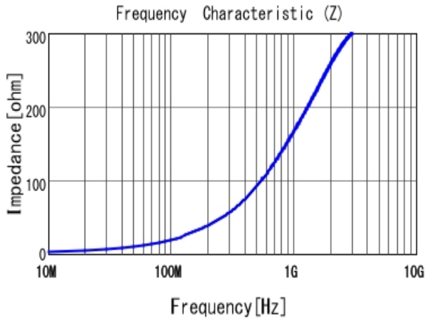
■ LQW18CA32NJ00 |Z|
