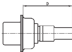
Einbaumaß
