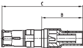
Buchsenkontakt
