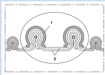
Klemmprofilschlauch, doppelagig (bis +170°C)
