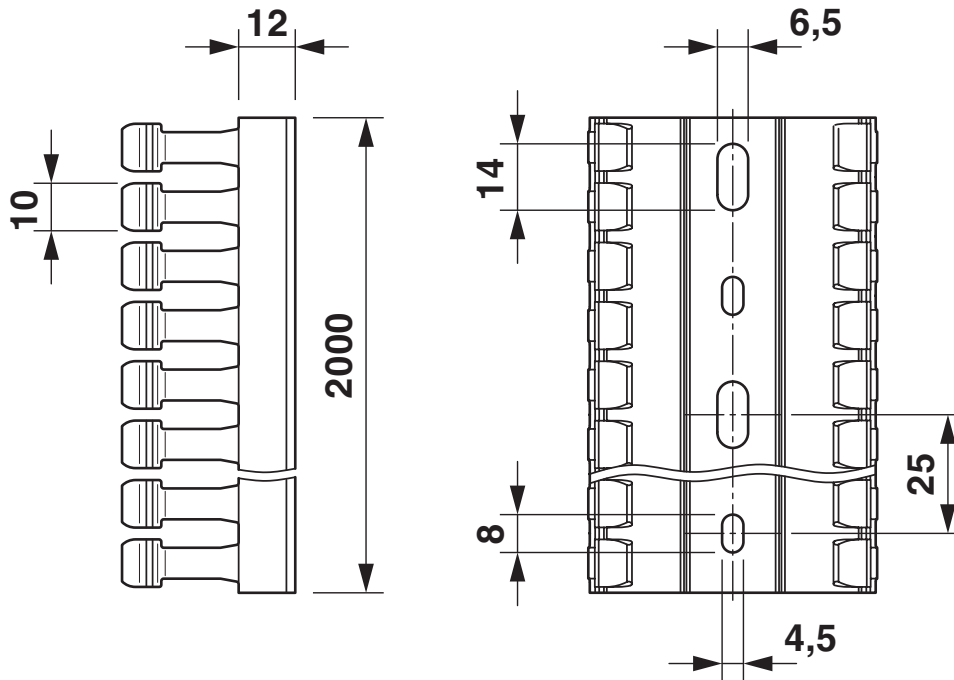
Maßzeichnung
